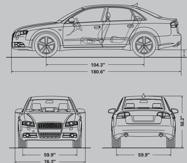
A4 Sedan
