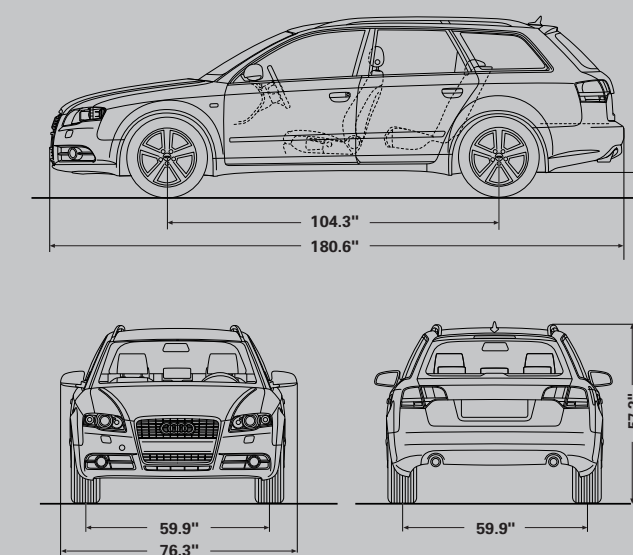
A4 Avant
